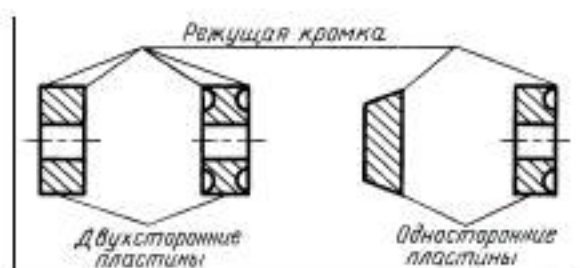
Режущая округленная кромка
