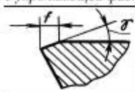
Режущая с упрочняющей фаской кромка
