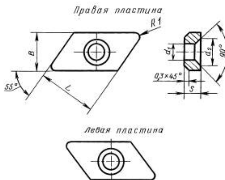
Размеры, мм
