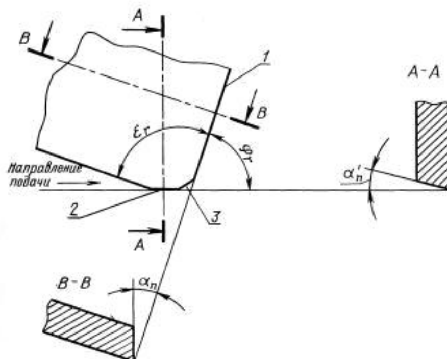
1 — главная режущая кромка; 2 — зачистная режущая фаска; 3 — переходная фаска Черт. 4
